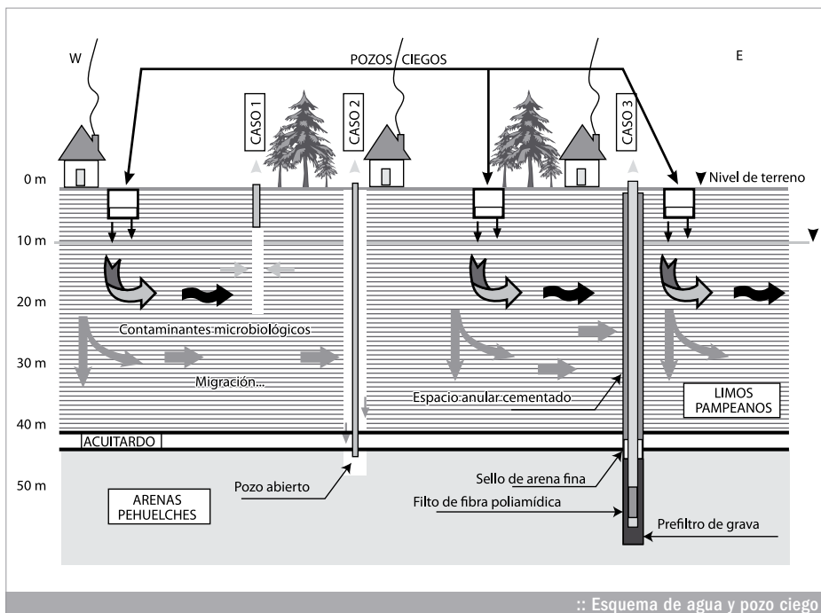
:: Esquema de agua y pozo ciego
